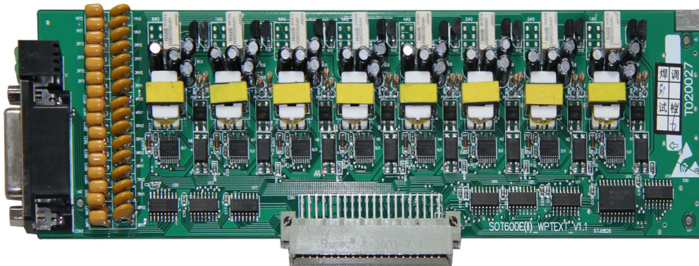
图 3-14 EXT 用户板
