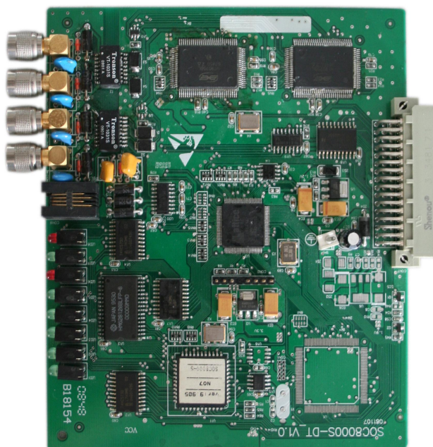
图 3-6 数字中继板
