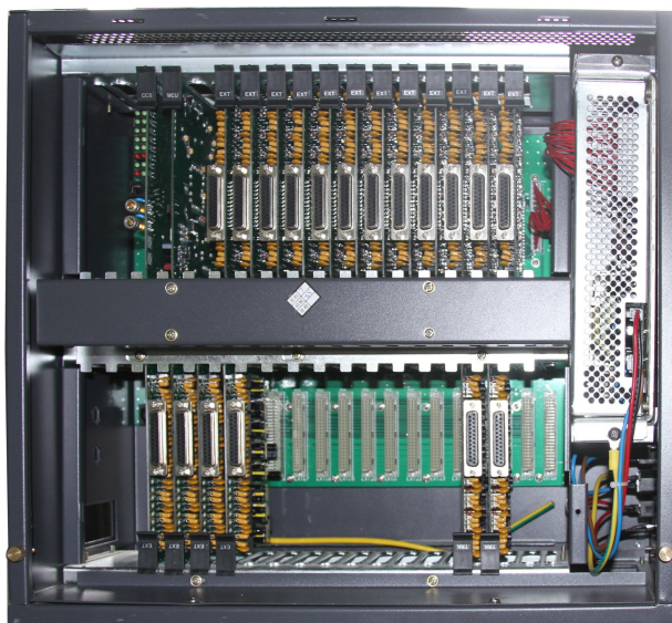
图 3-2 SOT600K 内部结构图
