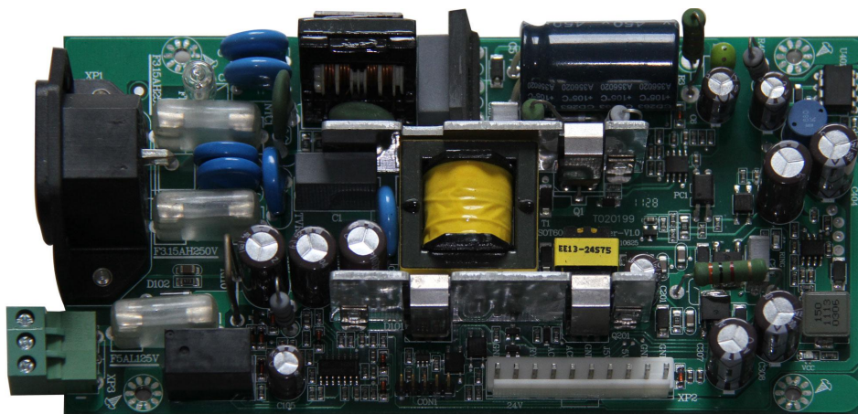
图 3-17 电源板
