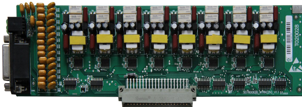
图 3-15 TRK 中继板
