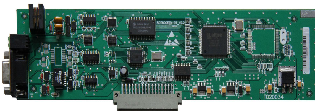
图 3-16 数字中继板
