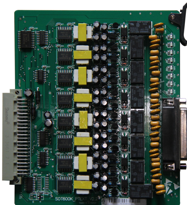
图 3-4 EXT 用户板
