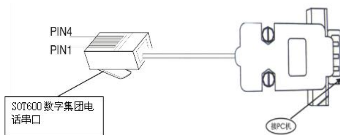
图 3-22 RS232 串口与电脑联机接口连接关系图
