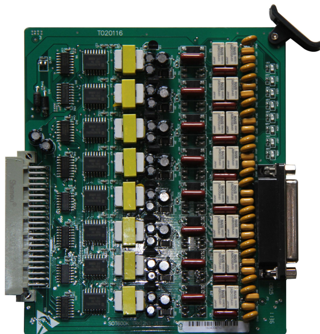
图 3-5 TRK 中继板
